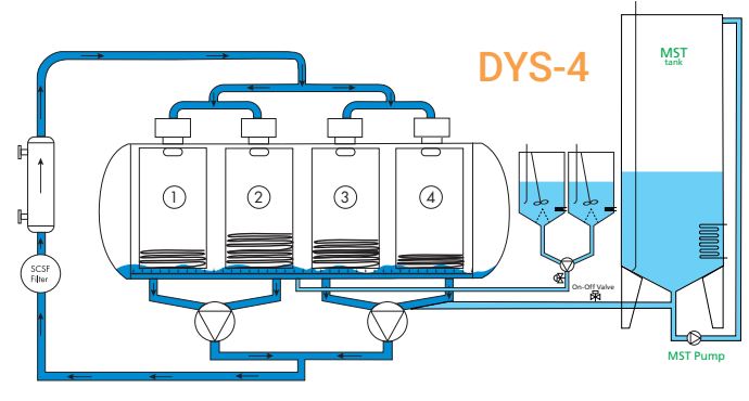
Versión con 4 cubas tejido y 2 bombas multisucción Version with 4 fabric deposits and 2 multisuction pumps
