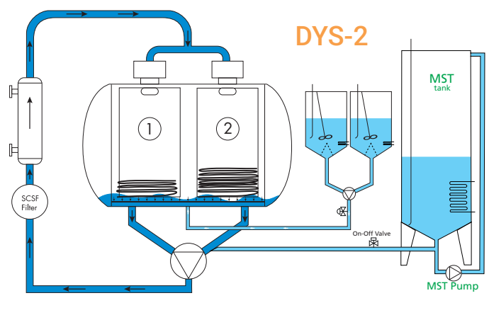
Versión con 2 cubas tejido y 1 bomba multisucción Version with 2 fabric deposits and 1 multisuction pump
